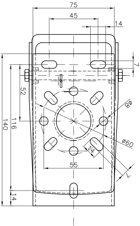
Vista A-A
